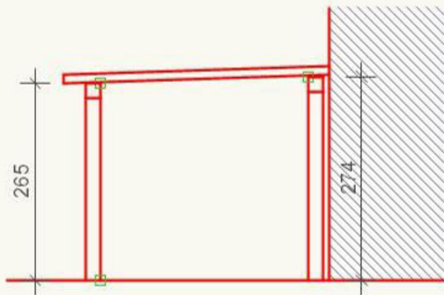
SEZIONE PORTICO "A"
