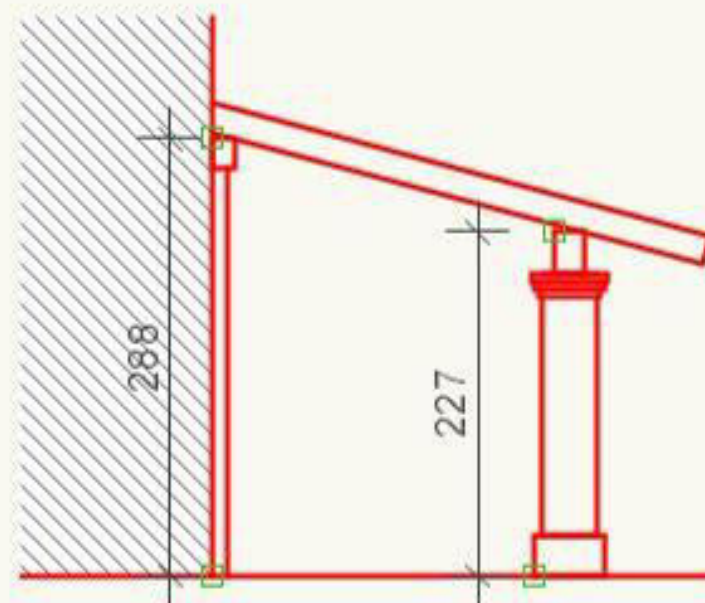
SEZIONE PORTICO "B"
